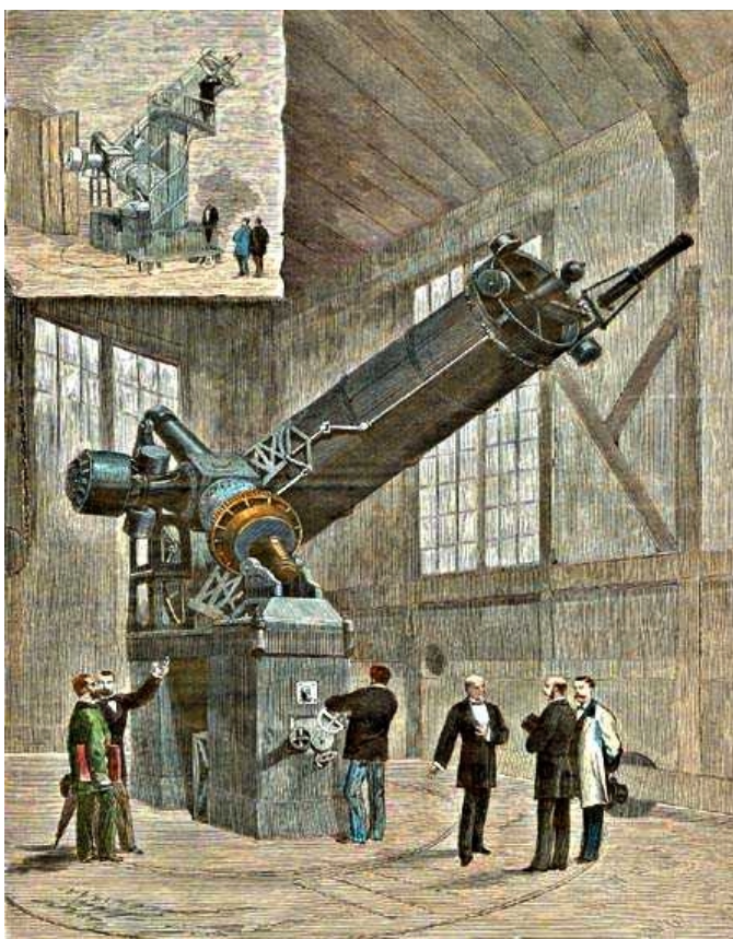
Fig. 2. Réception du télescope de 1,20-m dans les jardins de l'Observatoire de Paris le 16 septembre 1875 (Le monde illustré, 16 octobre 1875).
