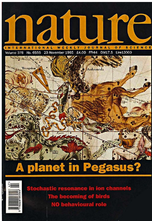
Fig. 3. Couverture de l'hebdomadaire anglais "Nature" du 23 novembre 1995 annonçant la découverte faite à l'OHP par les astronomes suisses Mayor et Queloz de la première exoplanète.
