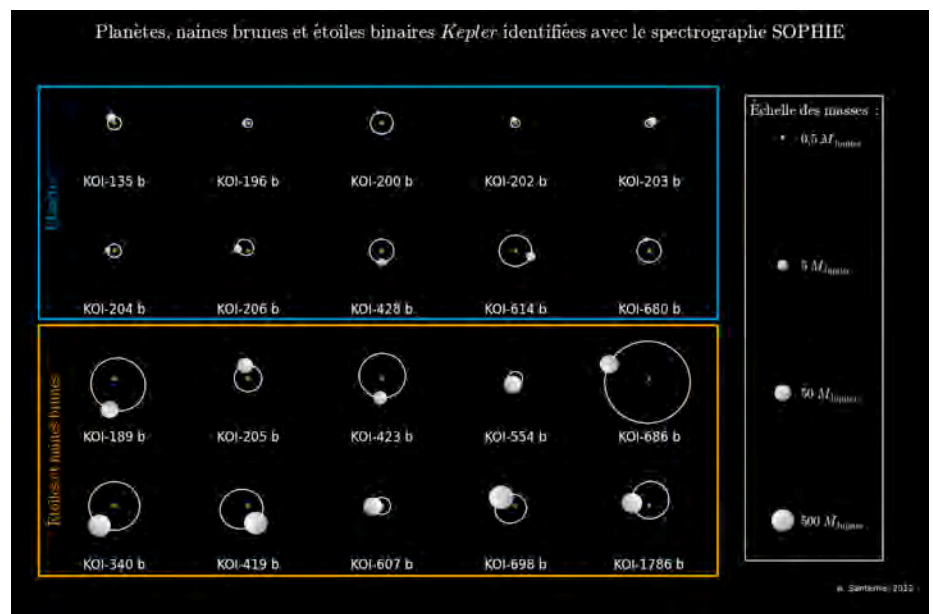
Planètes, naines brunes et étoiles binaires Kepler identifiées avec le spectrographe SOPHIE. La taille des objets est proportionnelle à leur masse. Une version animée est disponible à l'adresse : ftp://oamp.fr/pub/asanterne/kepler/PressRelease/
