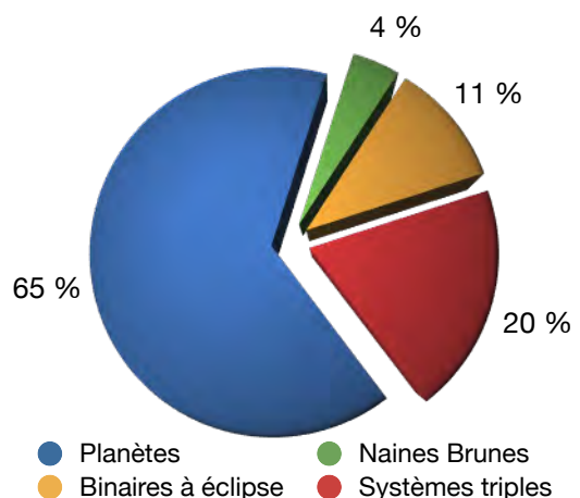
Nature des candidats-planètes Kepler déterminée grâce au spectrographe SOPHIE
